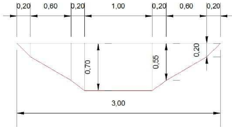
DIMENSIONS CARACTÉRISTIQUES DU PROFIL TYPE RECTILIGNE DU PROJET
