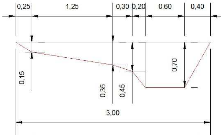
DIMENSIONS CARACTÉRISTIQUES DU PROFIL TYPE COURBE DU PROJET
